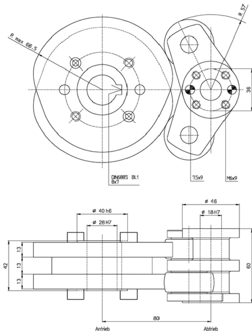
Fig 4: Einbausatz CF3-Pendelgetriebe Baureihe 80P
