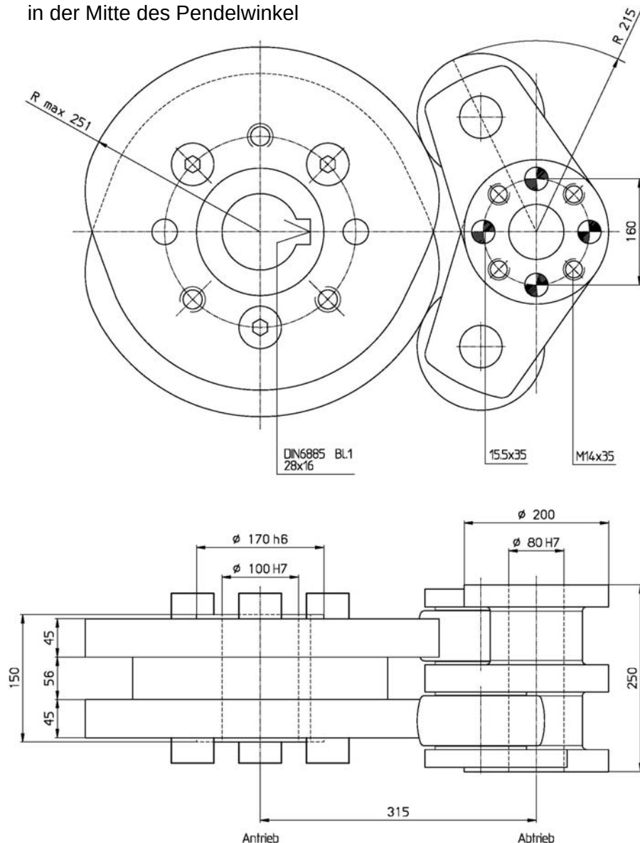
Fig 16: Einbausatz CF3-Pendelgetriebe Baureihe 315P
