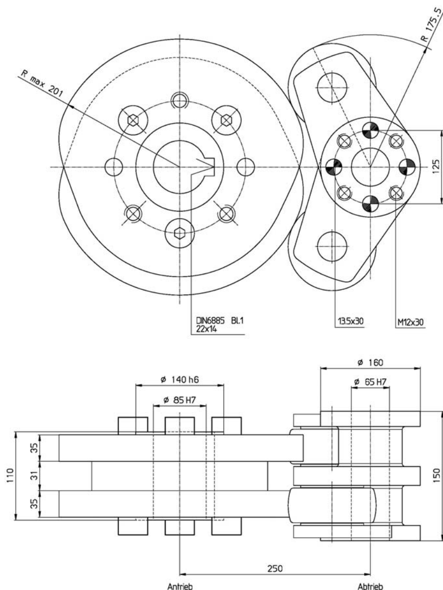
Fig 14: Einbausatz CF3-Pendelgetriebe Baureihe 250P
