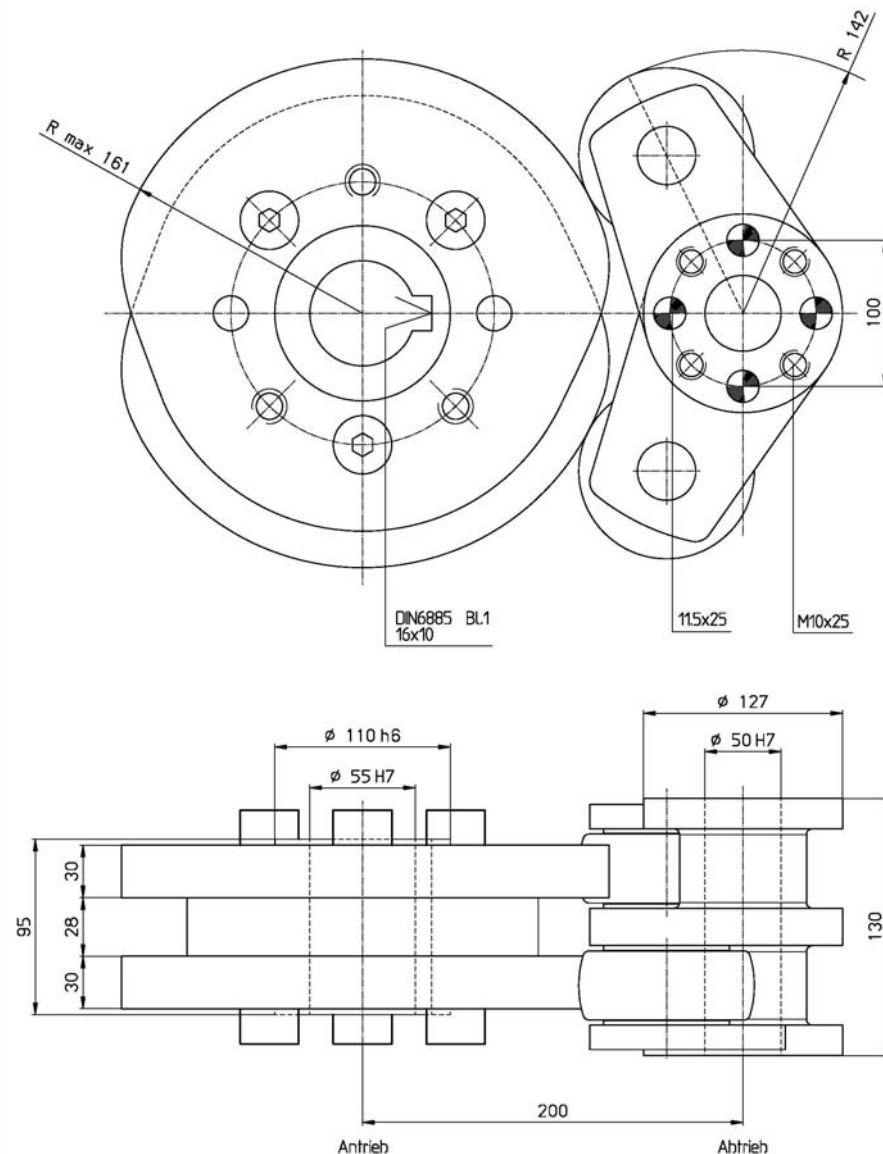
Fig 12: Einbausatz CF3-Pendelgetriebe Baureihe 200P
