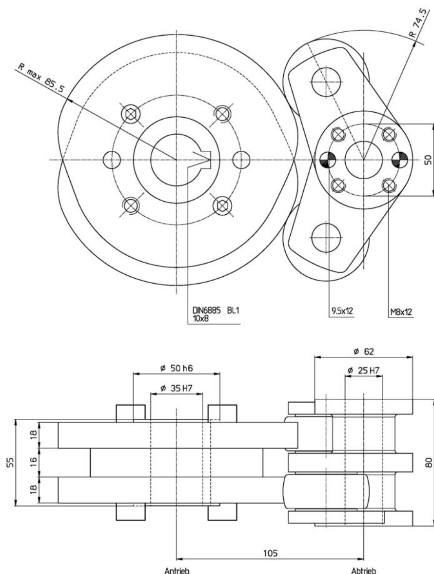
Fig 6: Einbausatz CF3-Pendelgetriebe Baureihe 105P
