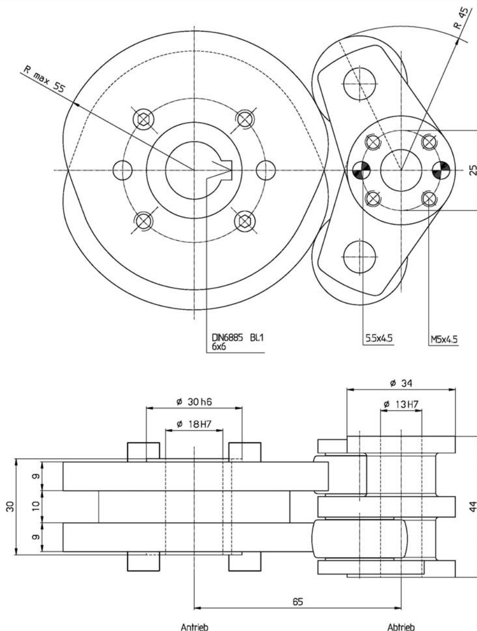
Fig 2: Einbausatz CF3-Pendelgetriebe Baureihe 65P
