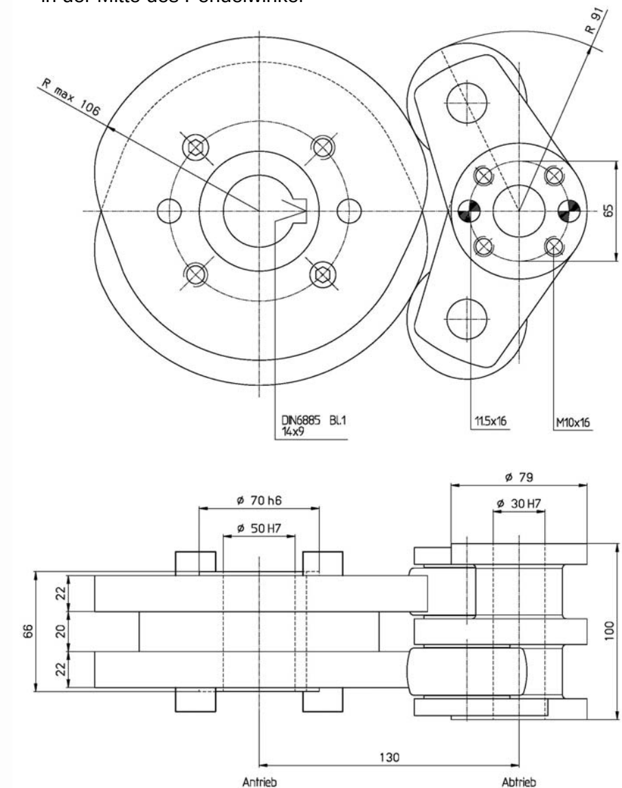
Fig 8: Einbausatz CF3-Pendelgetriebe Baureihe 130P
