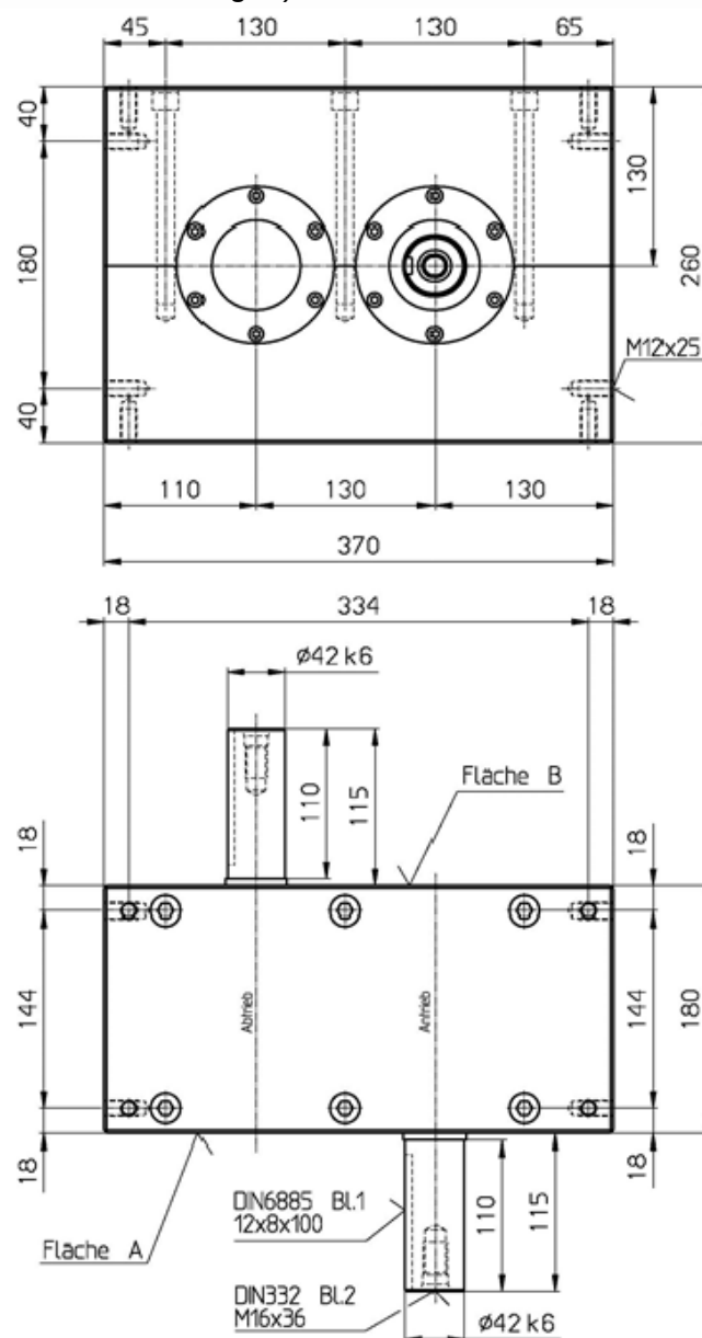
Fig 7: Gehäuseausführung CF3-Pendelgetriebe Baureihe 130P
