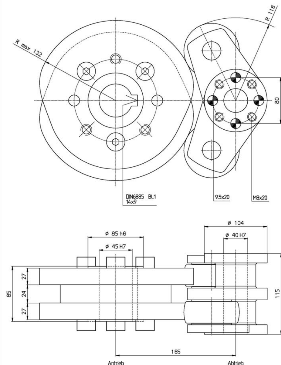
Fig 10: Einbausatz CF3-Pendelgetriebe Baureihe 165P
