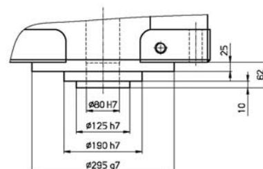
Fig 15: Gehäuseausführung CF3-Pendelgetriebe Baureihe 315P
