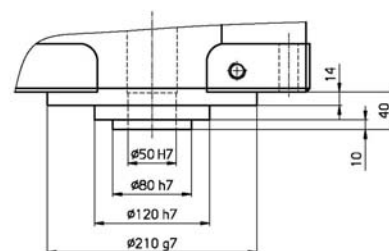
Fig 11: Gehäuseausführung CF3-Pendelgetriebe Baureihe 200P
