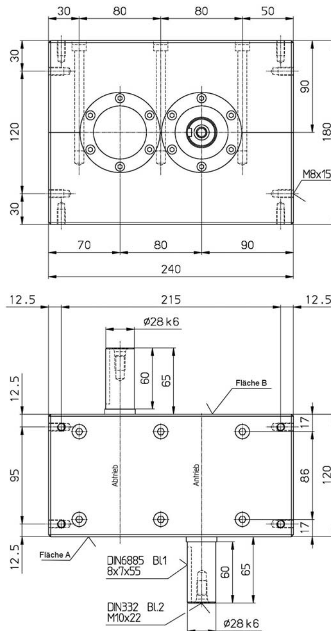
Fig 3: Gehäuseausführung CF3-Pendelgetriebe Baureihe 80P
